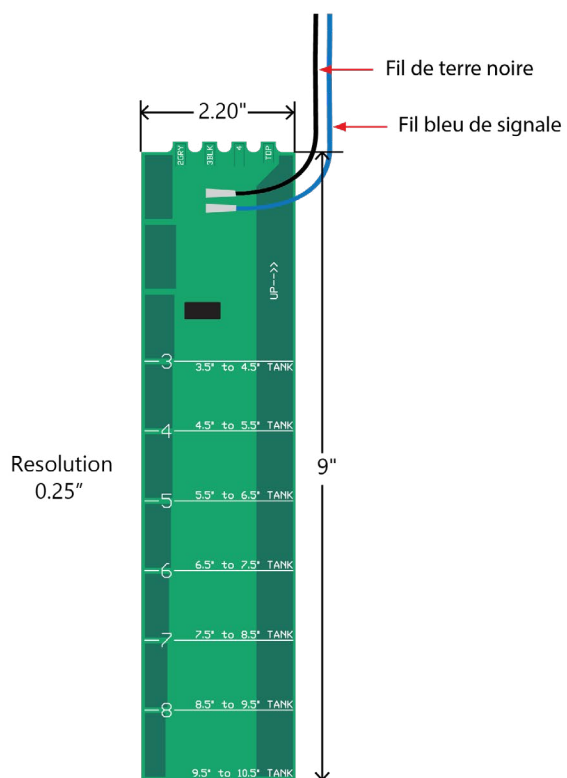
710-AR2 Transmetteur
